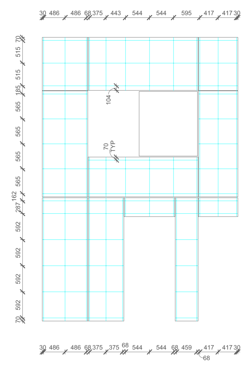
2 Façade B ÉCHELLE 1:50
