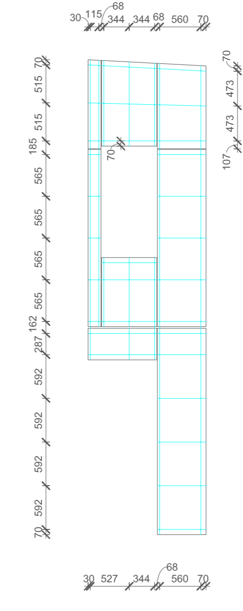
3 Façade C ÉCHELLE 1:50
