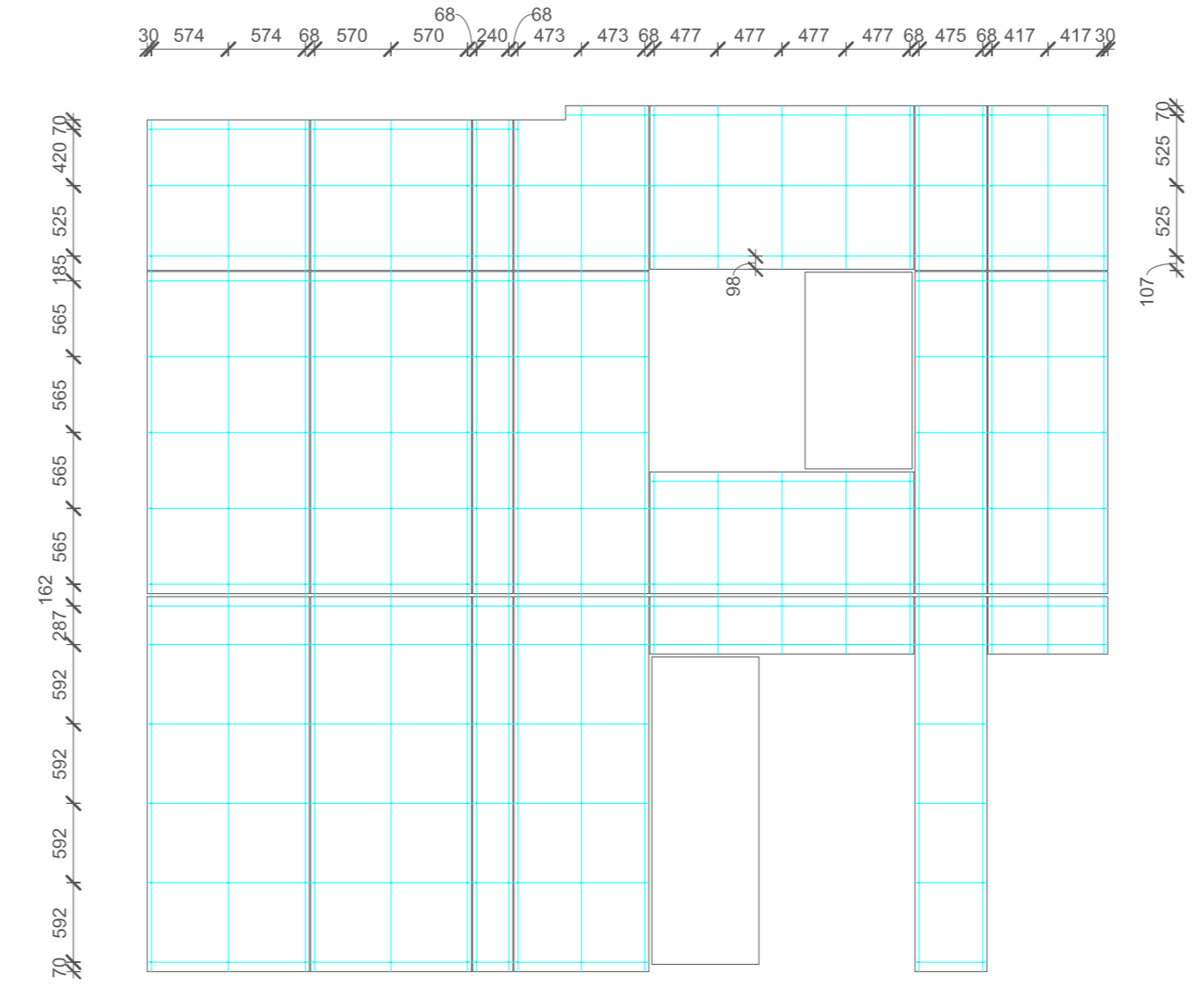
4 Façade D ÉCHELLE 1:50
